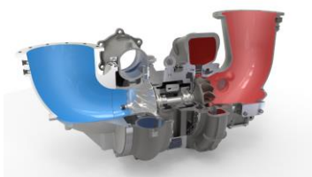
Querschnitt eines Turboladers der HPR-Serie.
